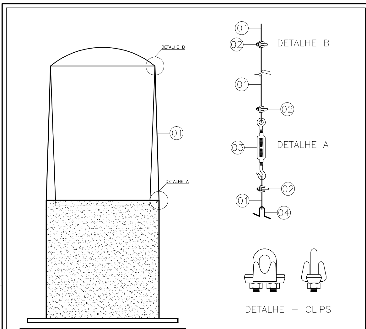
DETALHE FIXAÇÃO DOS TIRANTES – RAD – 5 A 20 M3
