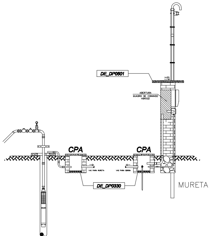
POÇO TUBULAR
